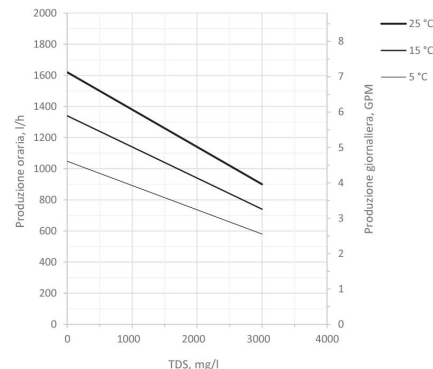
CAPACITÀ DI FLUSSO ENKISOFT MO24000 CON MEMBRANE XLE-4040
